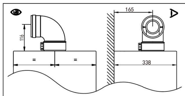
Присоединительные размеры при установке начального отвода 90° для модели 1.36F
