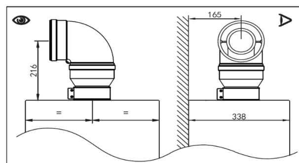
Присоединительные размеры при установке адаптера для перехода на систему 80/125 мм и отвода 90° для модели 1.36F
