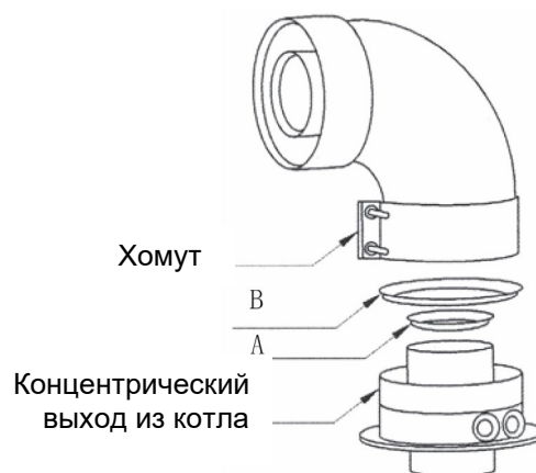
Диафрагмы для моделей 31F, 1.31F
