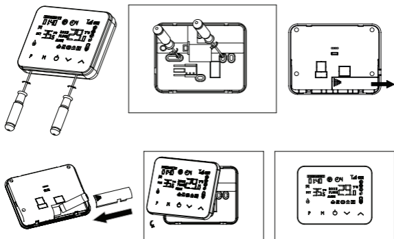
Рис.3 Установка терморегулятора на стену.
