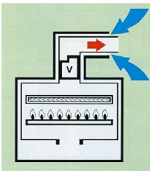
Забор воздуха и отвод продуктов сгорания по коаксиальным трубам
